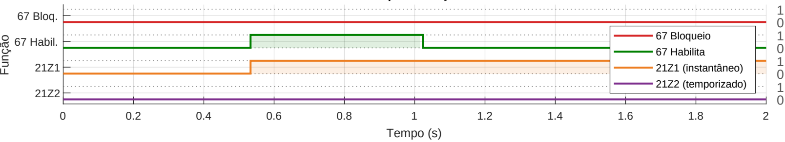
Status de trip das funções 21/67
